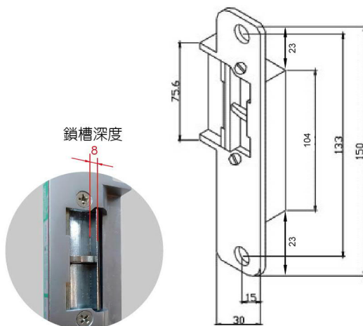
尺寸圖
